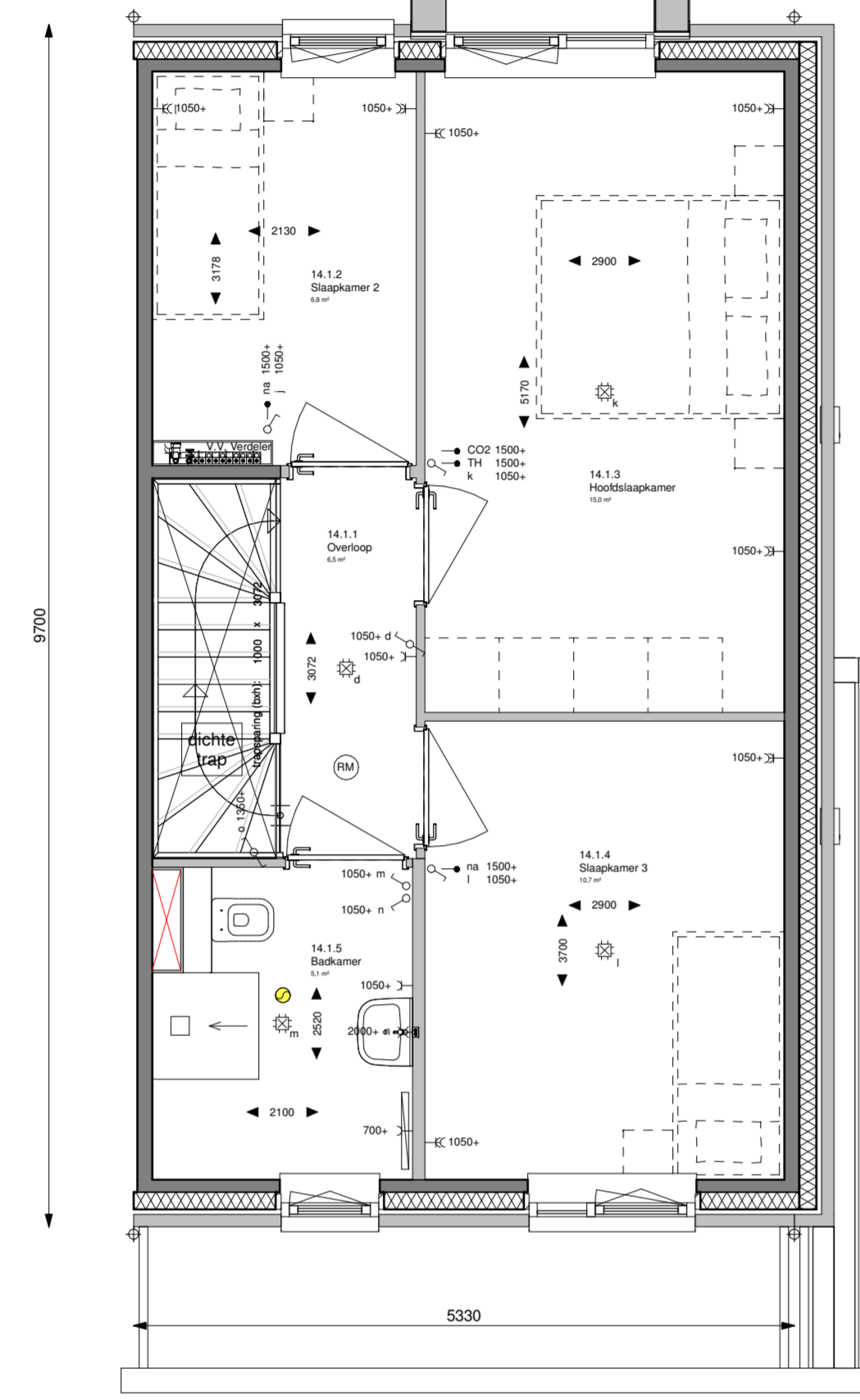
EERSTE VERDIEPING BASIS schaal 1:50
