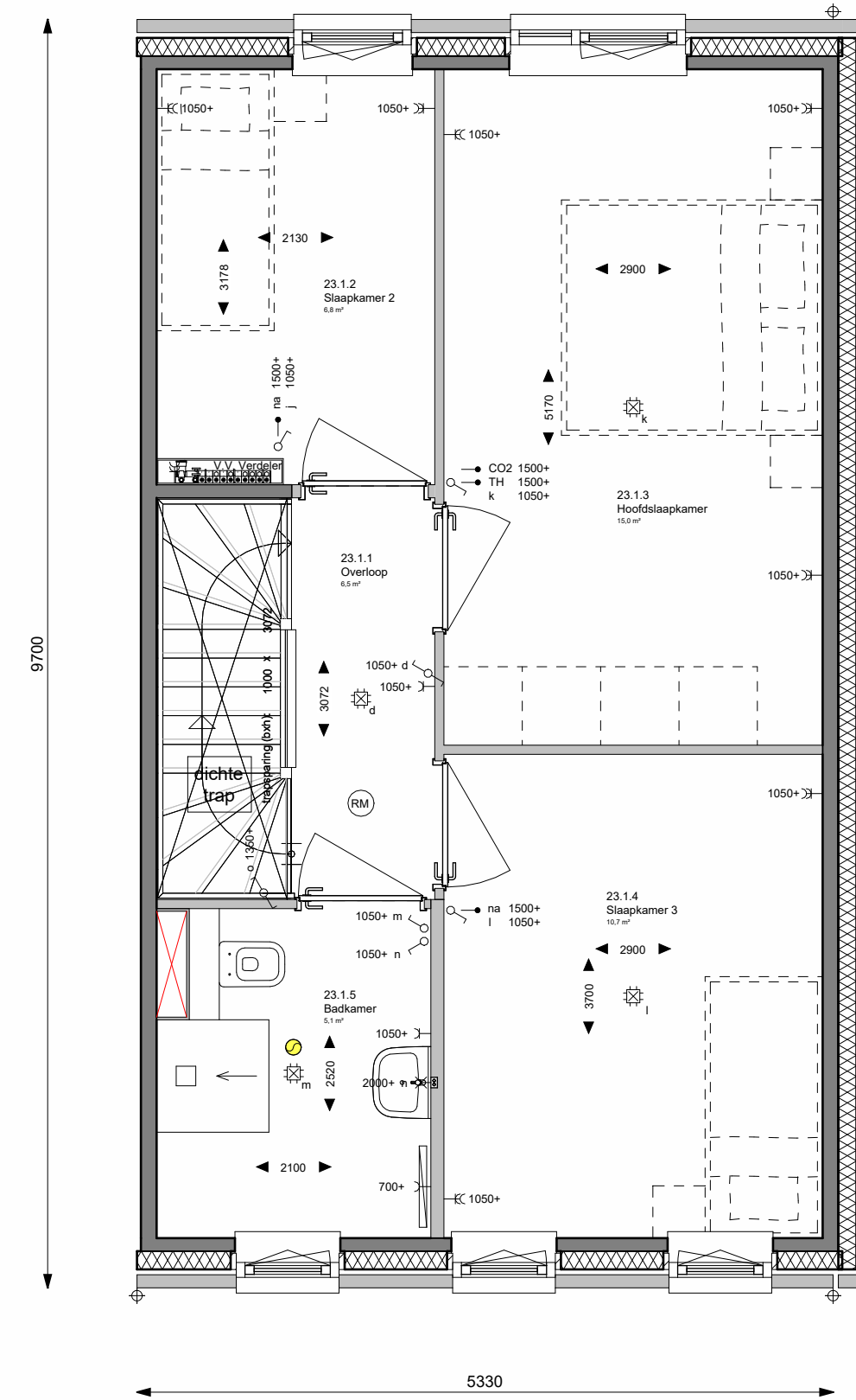
EERSTE VERDIEPING BASIS schaal 1:50
