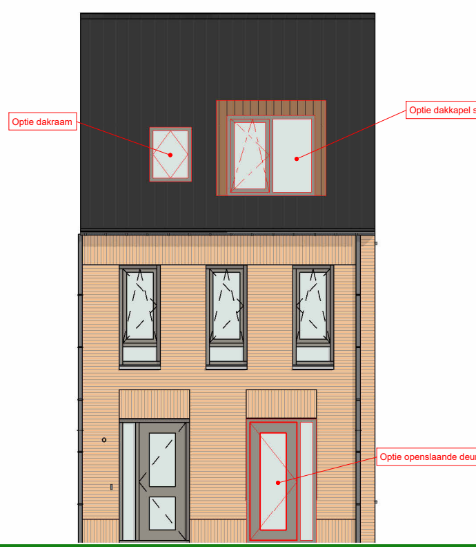
VOORGEVEL OPTIES Schaal 1:100
