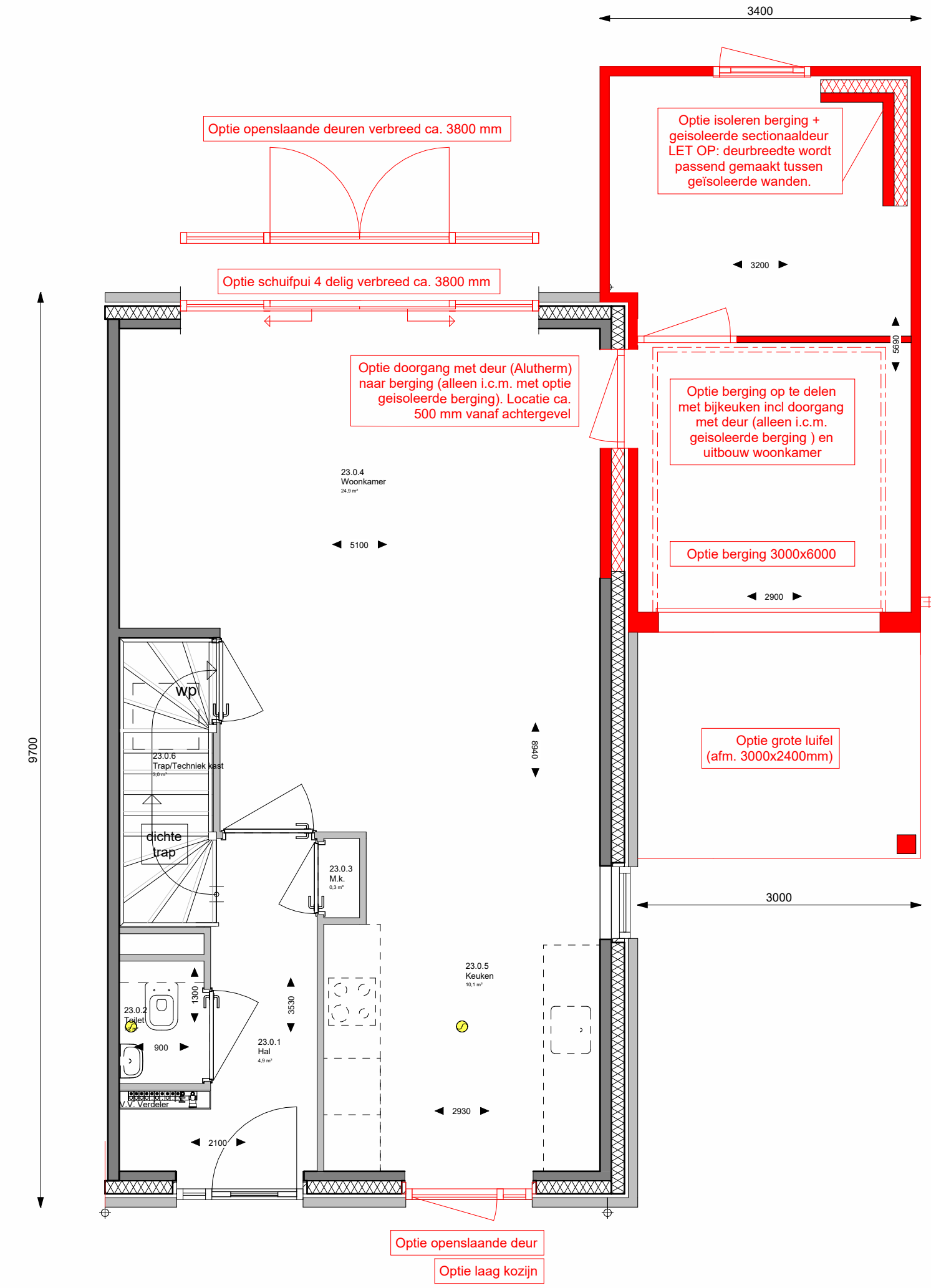
BEGANE GROND OPTIES schaal 1:50
