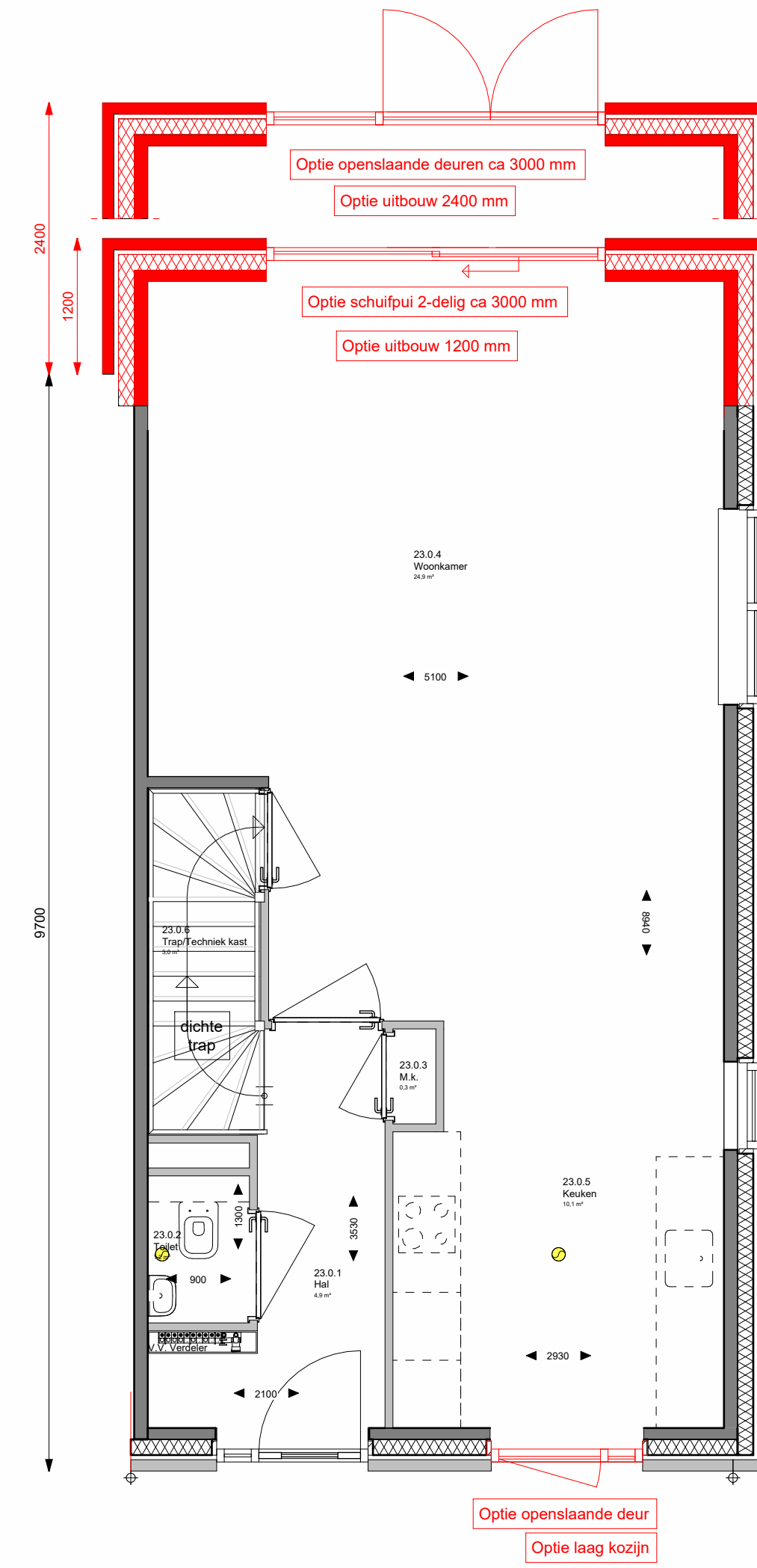
BEGANE GROND OPTIES schaal 1:50
