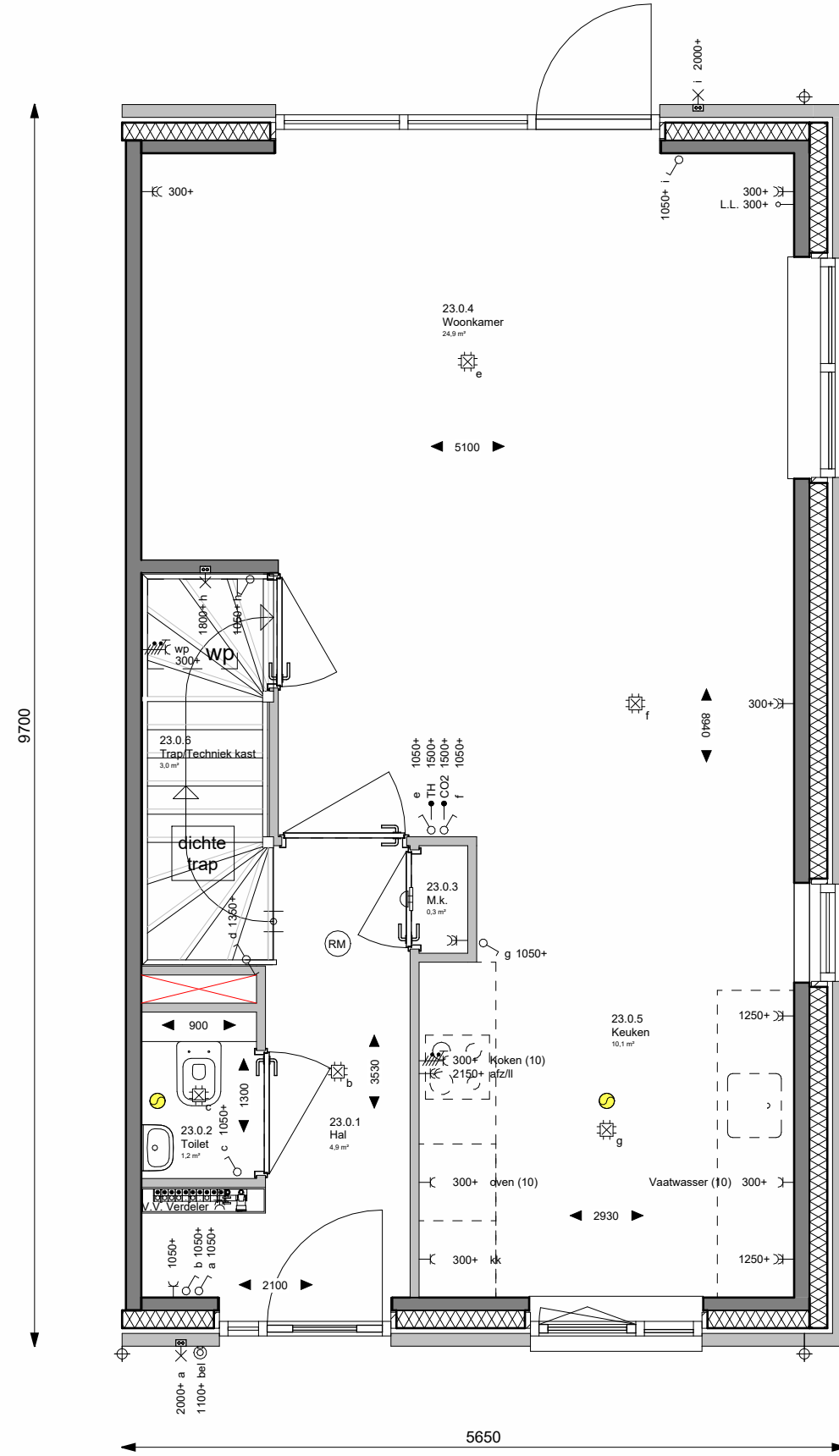
BEGANE GROND BASIS schaal 1:50
