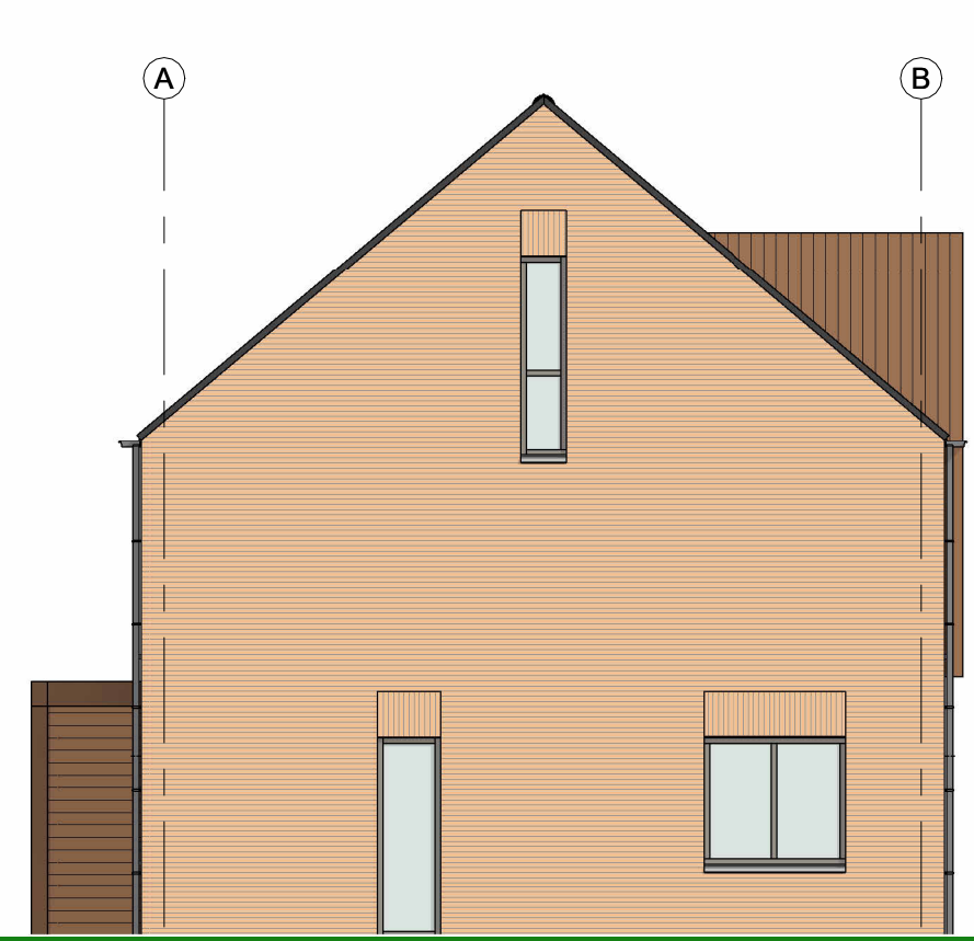
RECHTERGEVEL BASIS schaal 1:100
