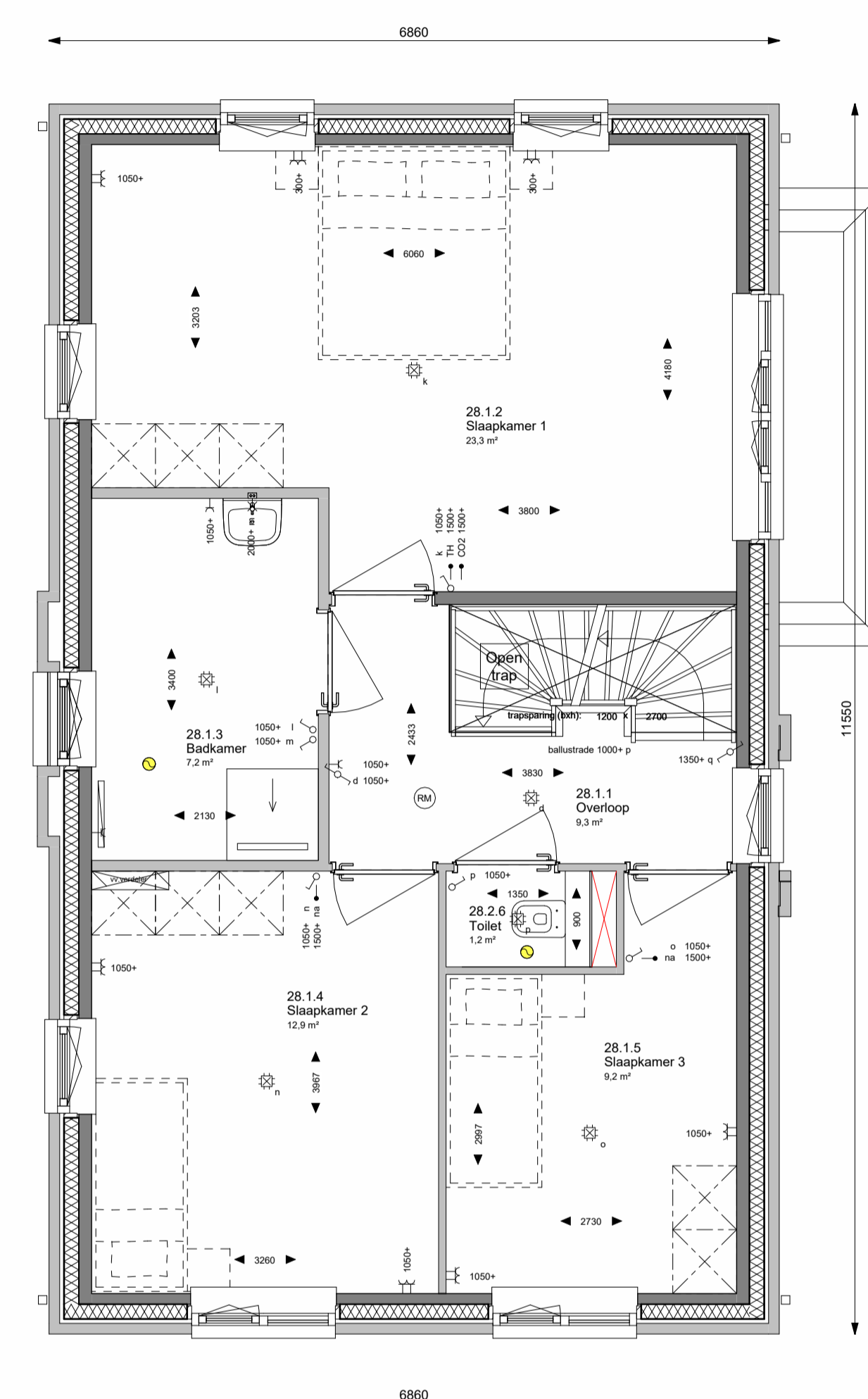
EERSTE VERDIEPING BASIS schaal 1:50
