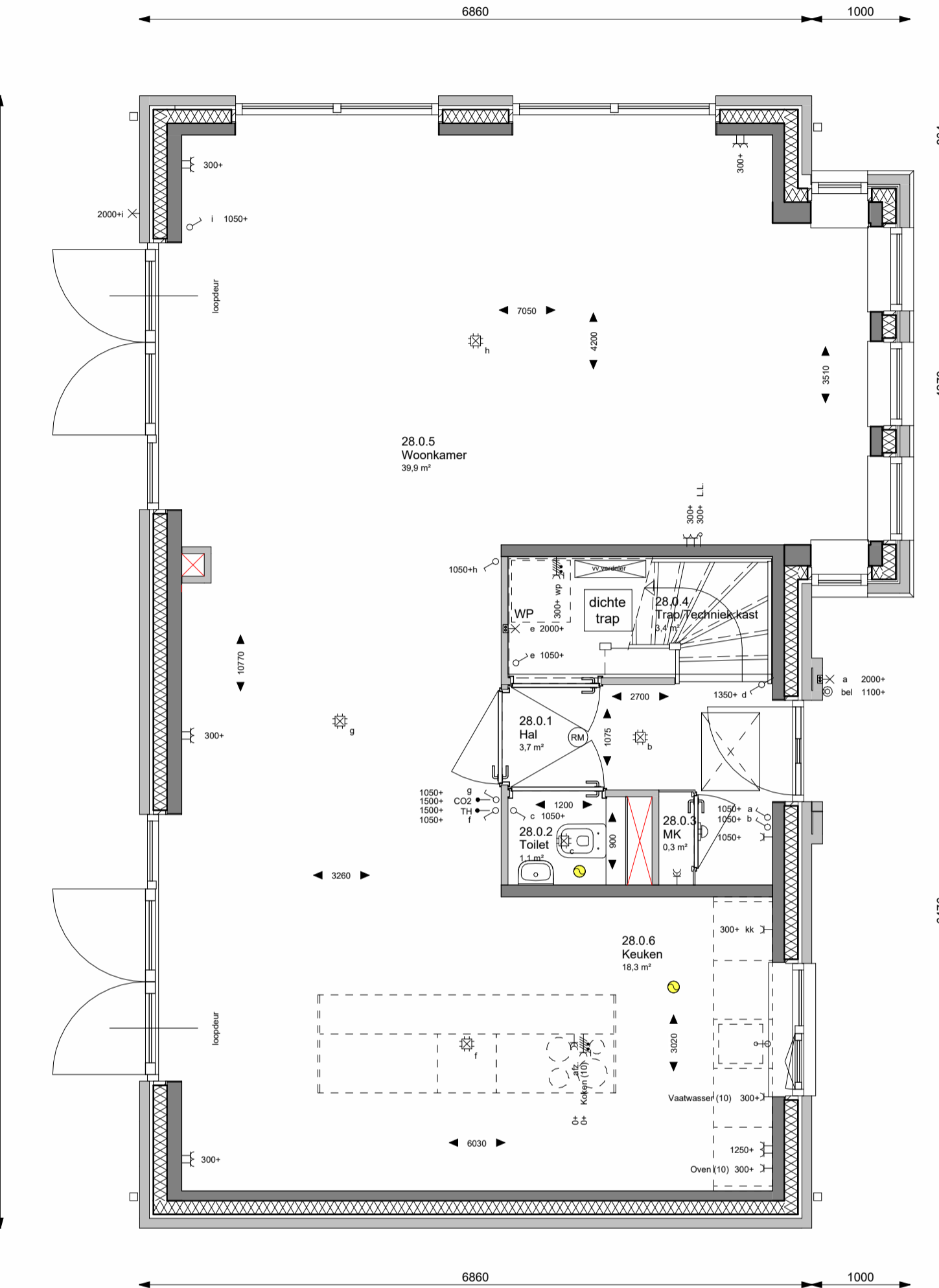
BEGANE GROND BASIS schaal 1:50
