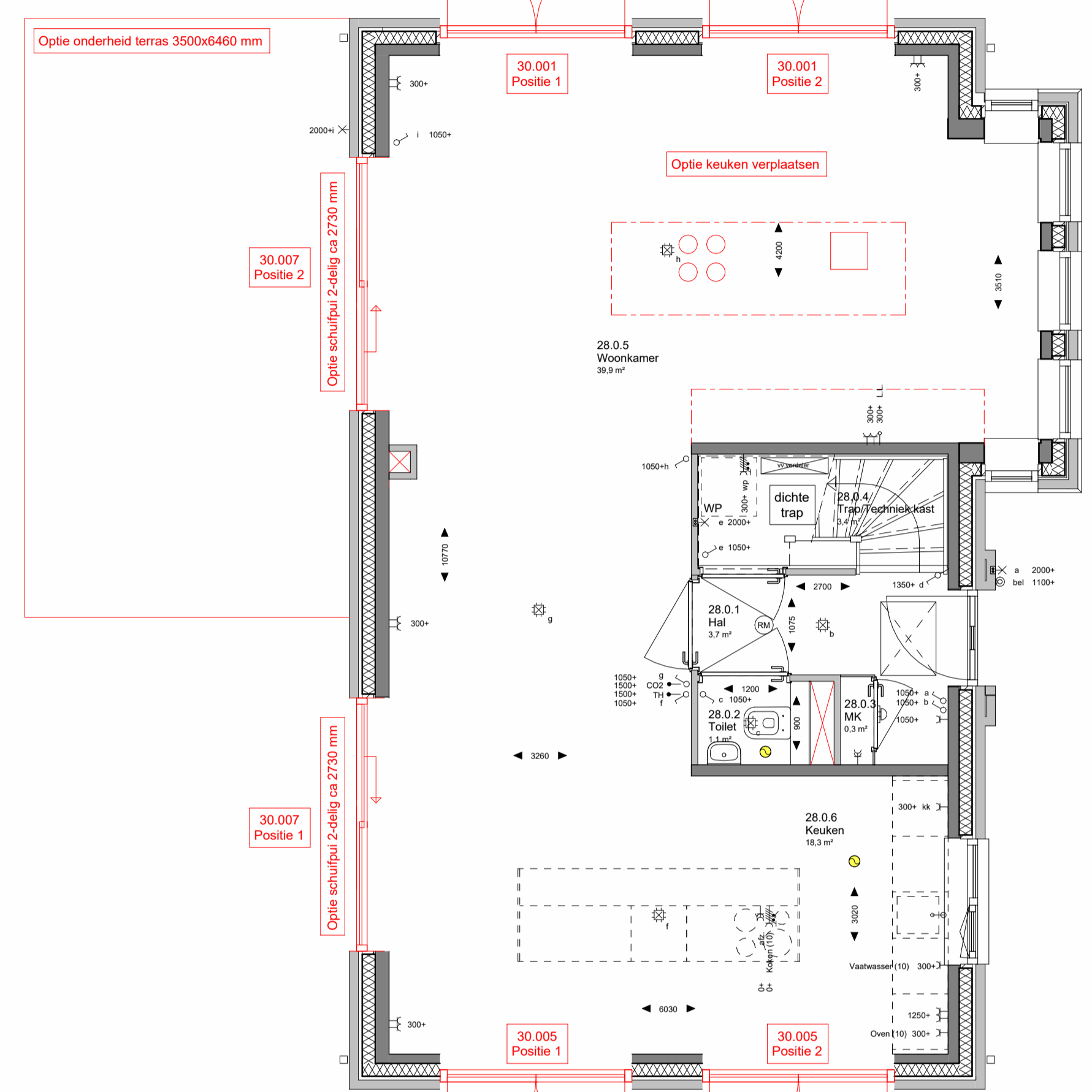
BEGANE GROND OPTIES schaal 1:50
