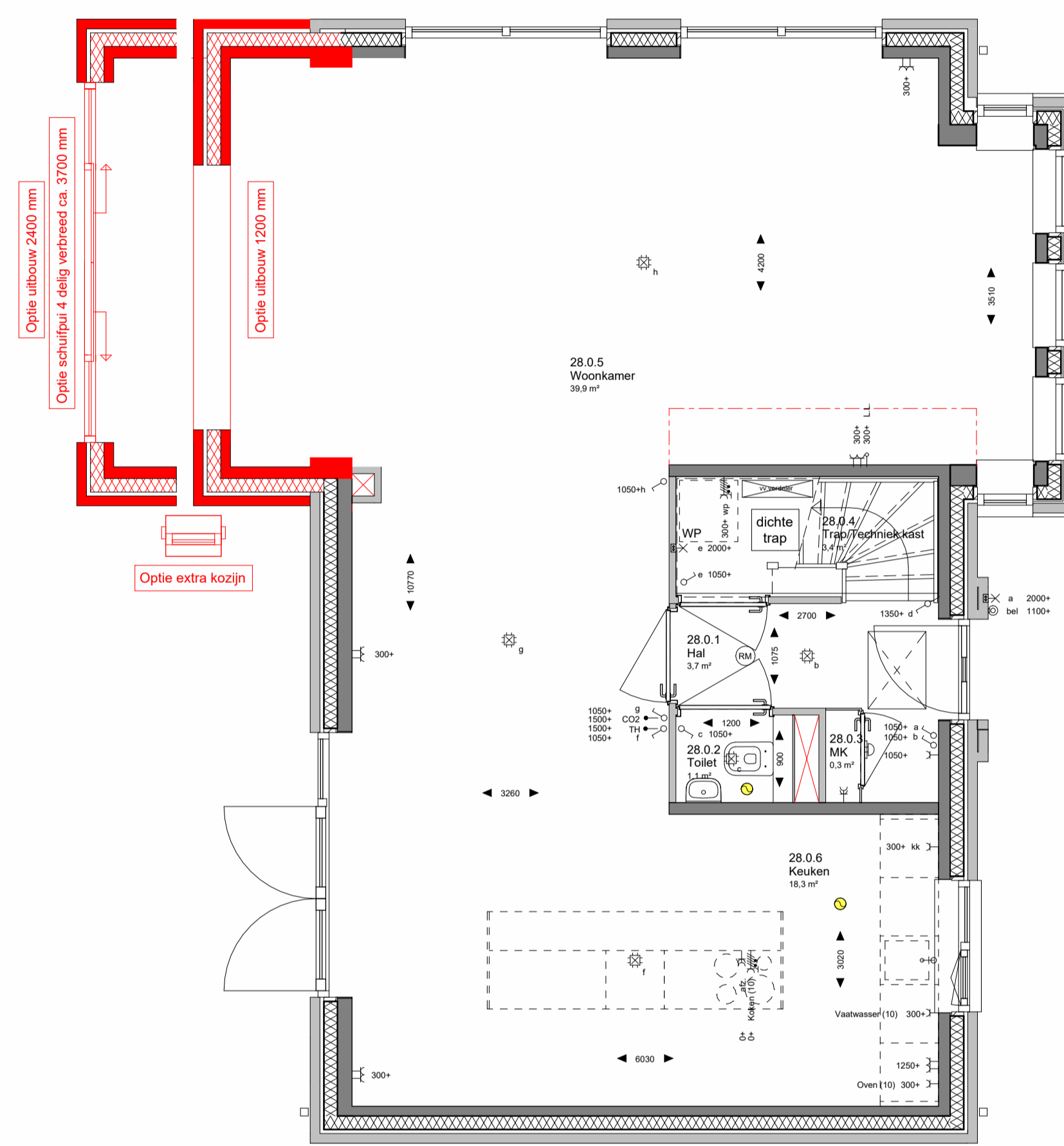
BEGANE GROND OPTIES schaal 1:50
