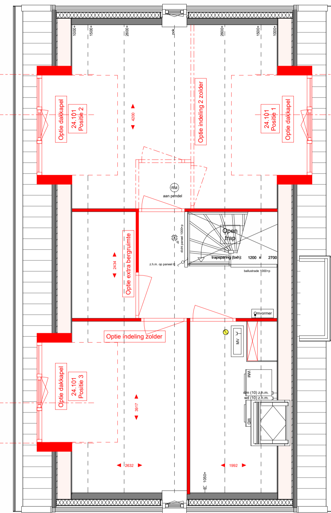
ZOLDER VERDIEPING OPTIES schaal 1:50
