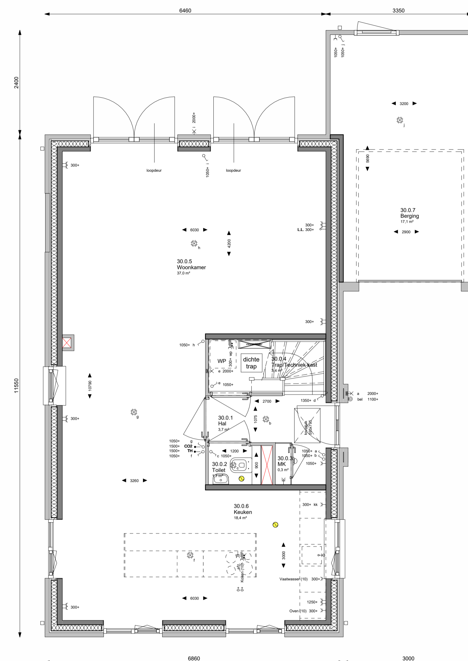
BEGANE GROND BASIS schaal 1:50
