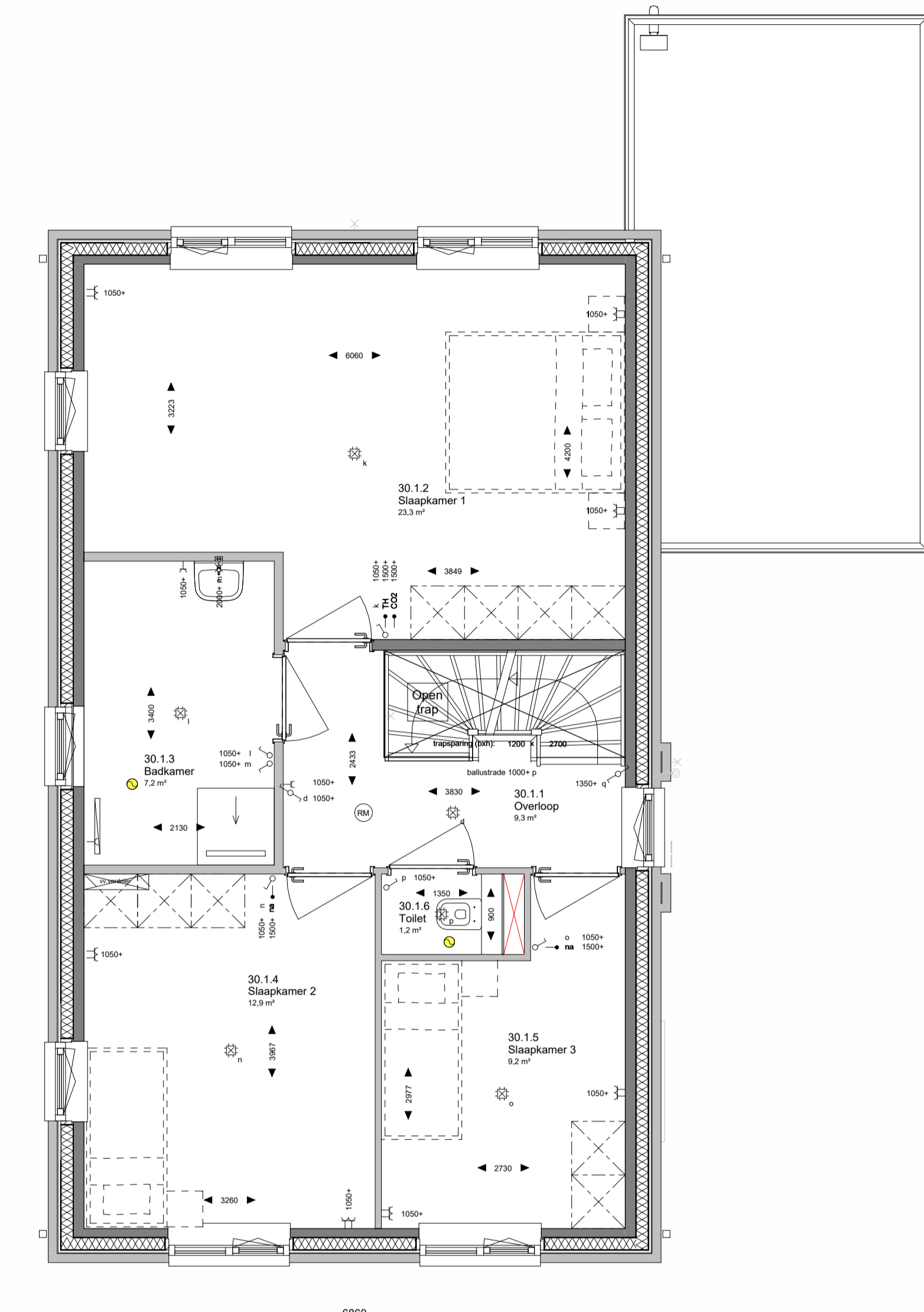
EERSTE VERDIEPING BASIS schaal 1:50
