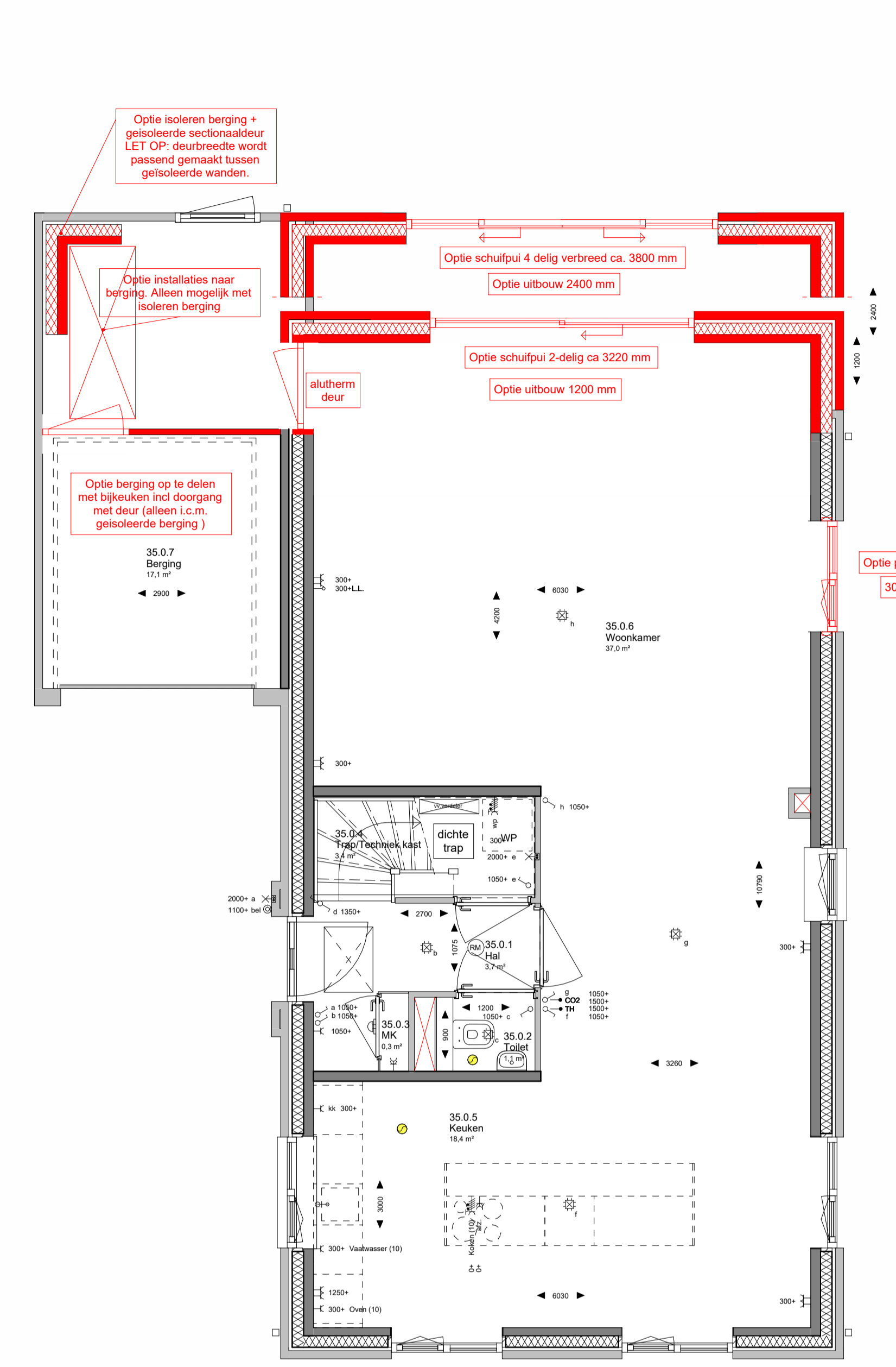
BEGANE GROND OPTIES schaal 1:50
