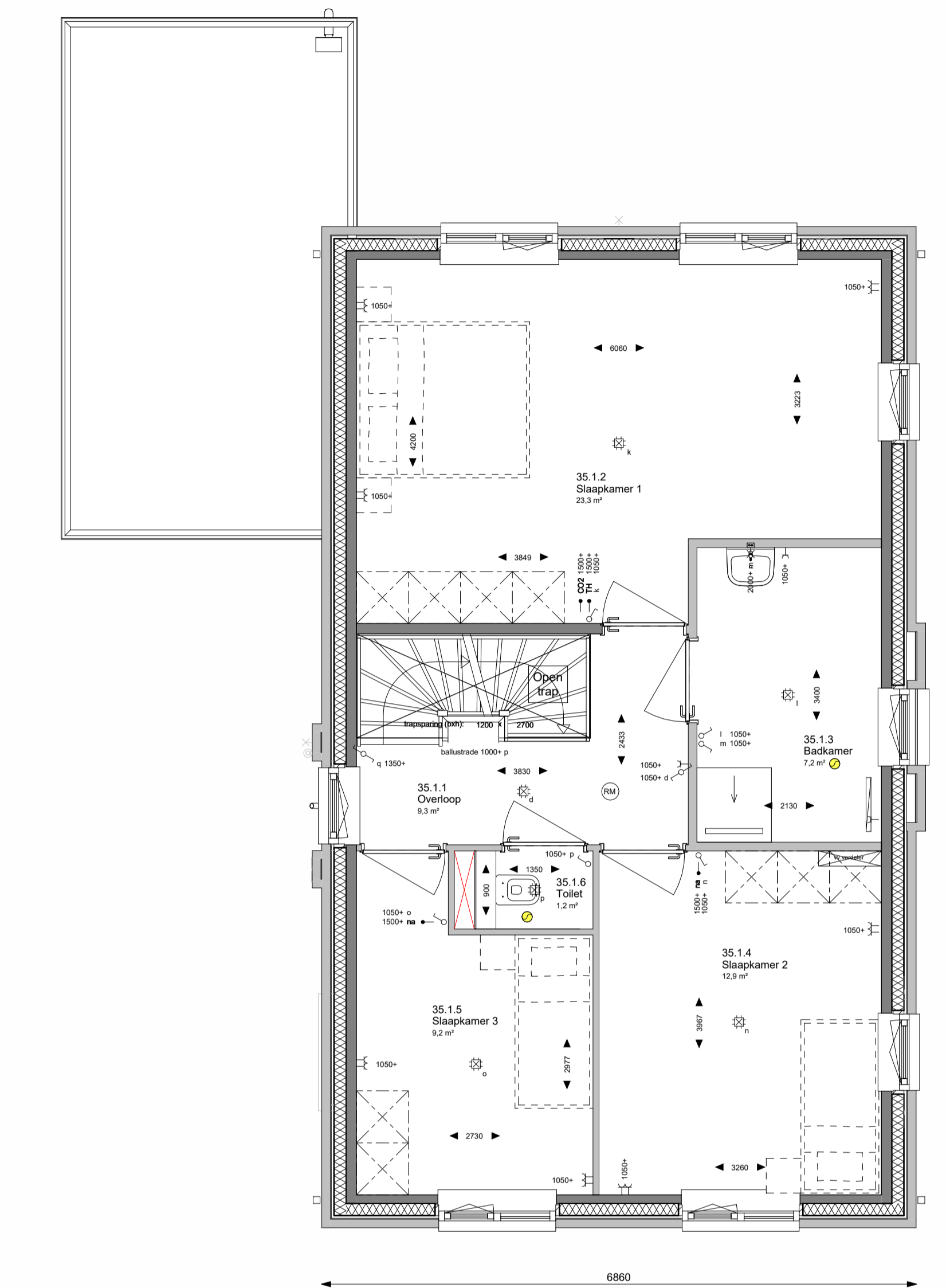
EERSTE VERDIEPING BASIS schaal 1:50
