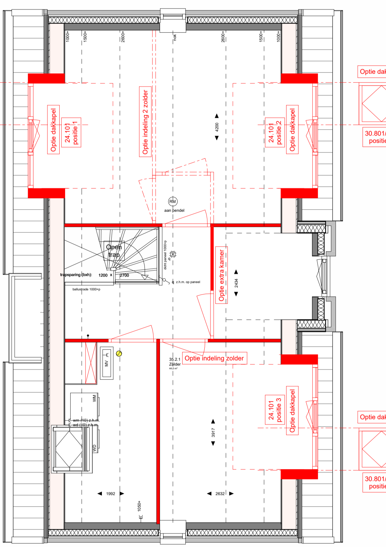
ZOLDER VERDIEPING OPTIES schaal 1:50
