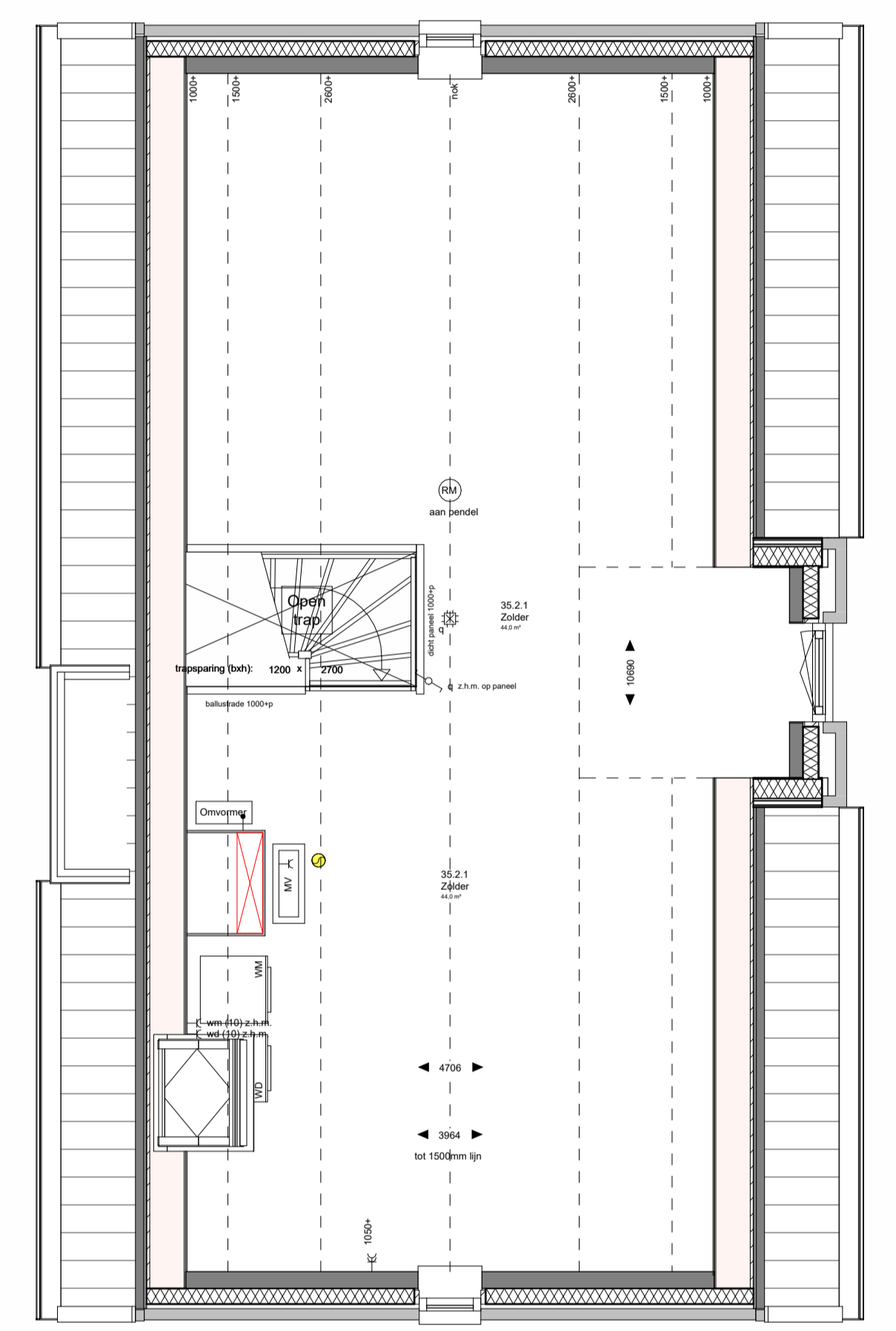
ZOLDER VERDIEPING BASIS schaal 1:50
