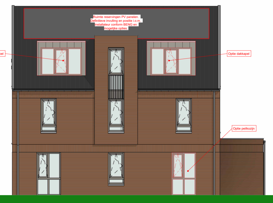
RECHTERGEVEL OPTIES Schaal 1:100
