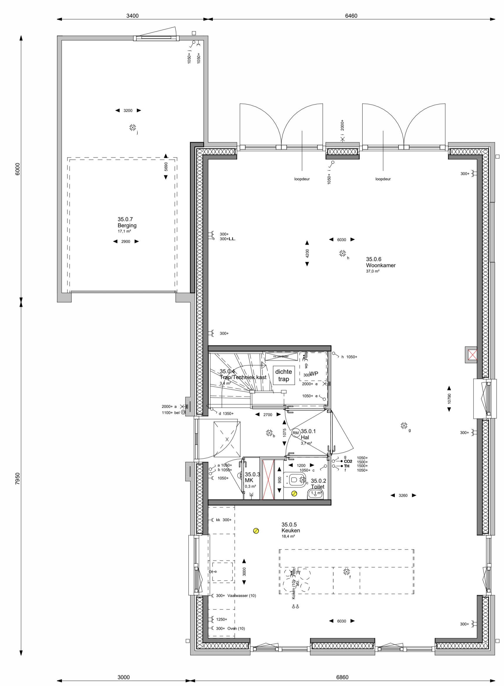
BEGANE GROND BASIS schaal 1:50
