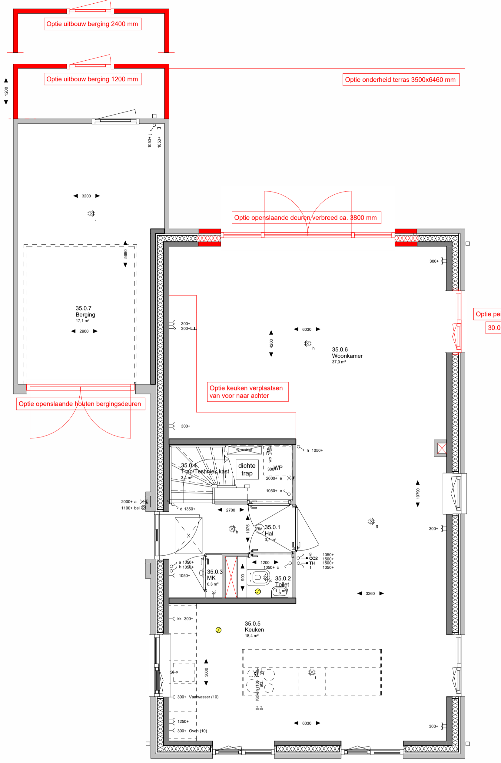
BEGANE GROND OPTIES schaal 1:50
